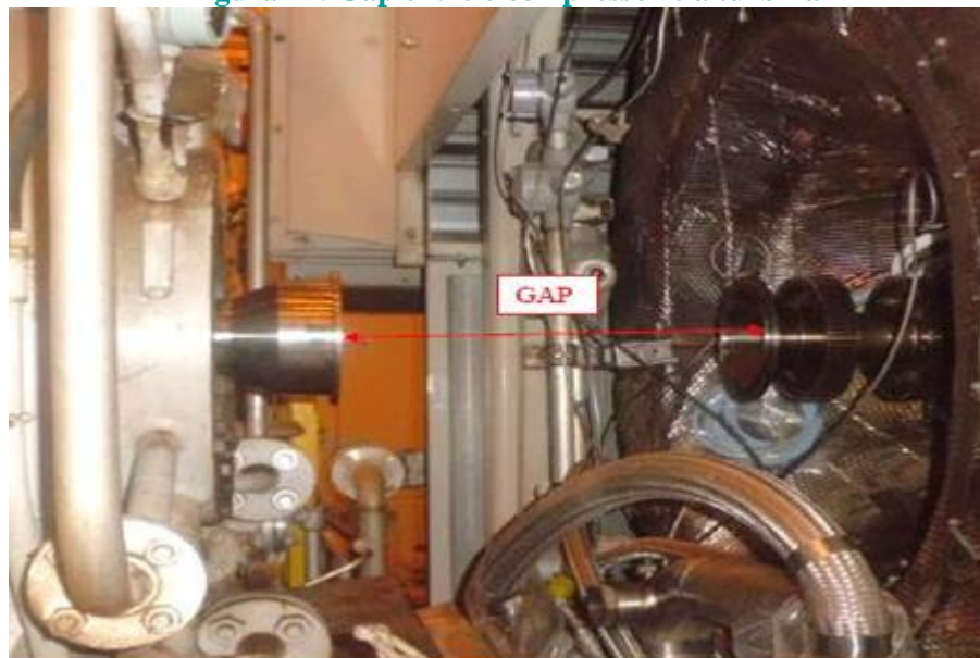
Figura 12: Gap entre o compressor e a turbina
