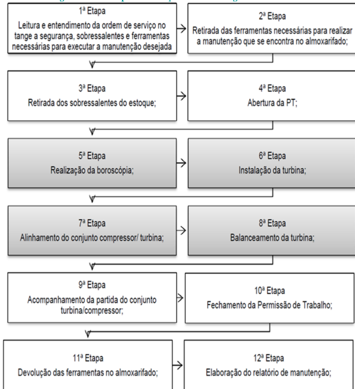
Figura 3: Roteiro para instalação da turbina a gás Solar Taurus 60
